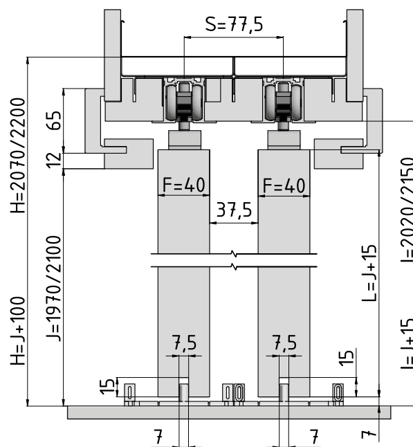
Horizontální řez pouzdra NORMA UNIBOX s dřevěným dveřním křídlem tloušťky 40 mm
