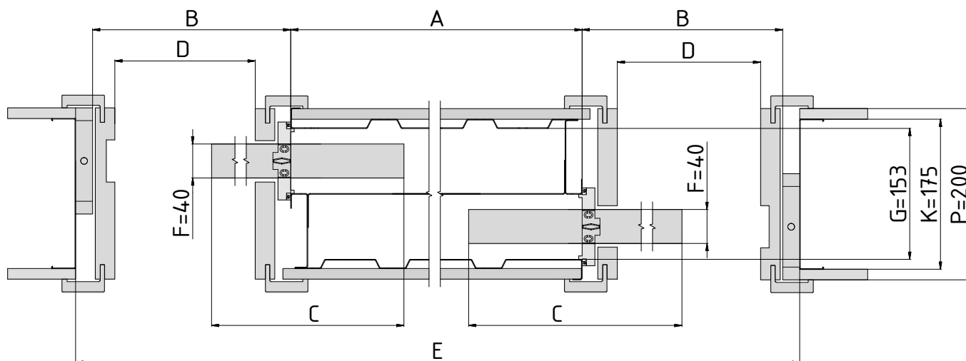
Vertikální řez pouzdra NORMA UNIBOX s dřevěným dveřním křídlem tloušťky 40 mm
