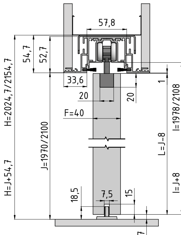
Vertikální řez pouzdra AKTIVE II STANDARD s dřevěným dveřním křídlem tloušťky 40 mm
