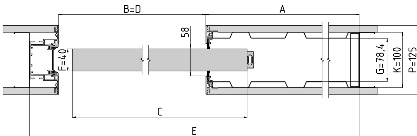
Horizontální řez pouzdra AKTIVE II STANDARD s dřevěným dveřním křídlem tloušťky 40 mm
